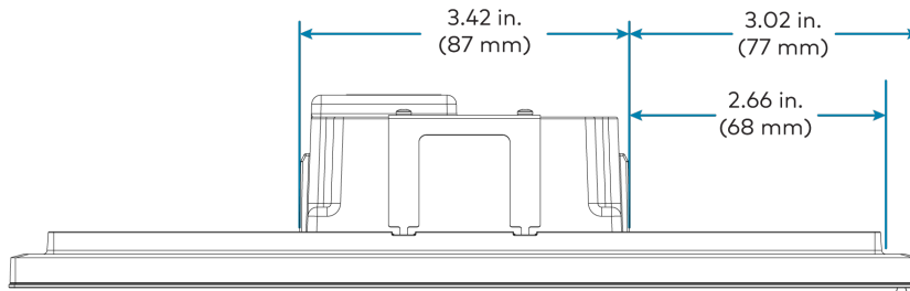
Touch Screen (TSW-1070-B-S-T-V )
